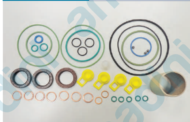
Kit universal/Universal kit CP1, CP3 0 445 020 *** 018/023/053/208
