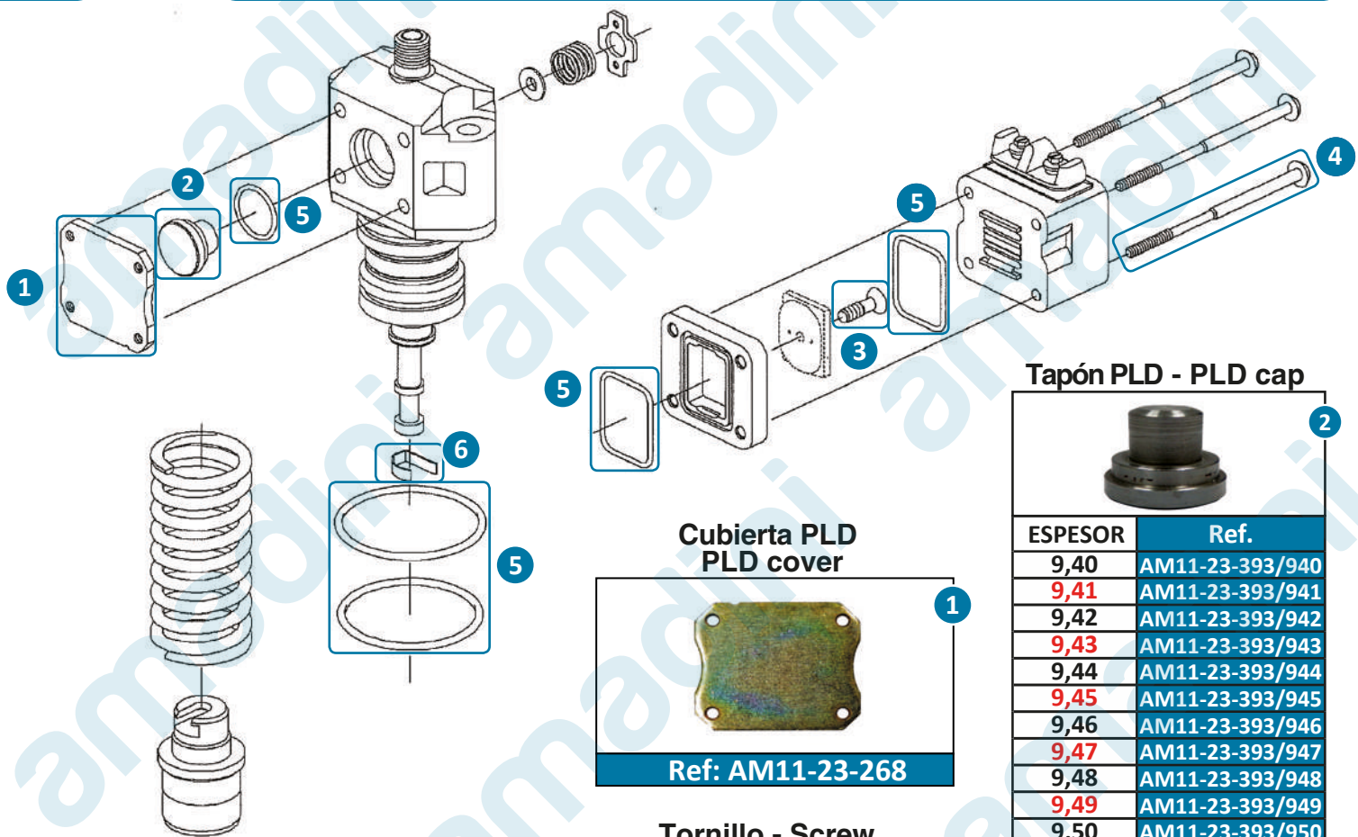
Tornillo - Screw
