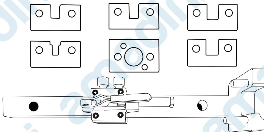
Ref: AM02-21-001 HERRAMIENTA DE MONTAJE - DESMONTAJE DEL INYECTOR
